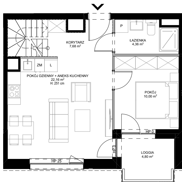
kondygnacja K3
