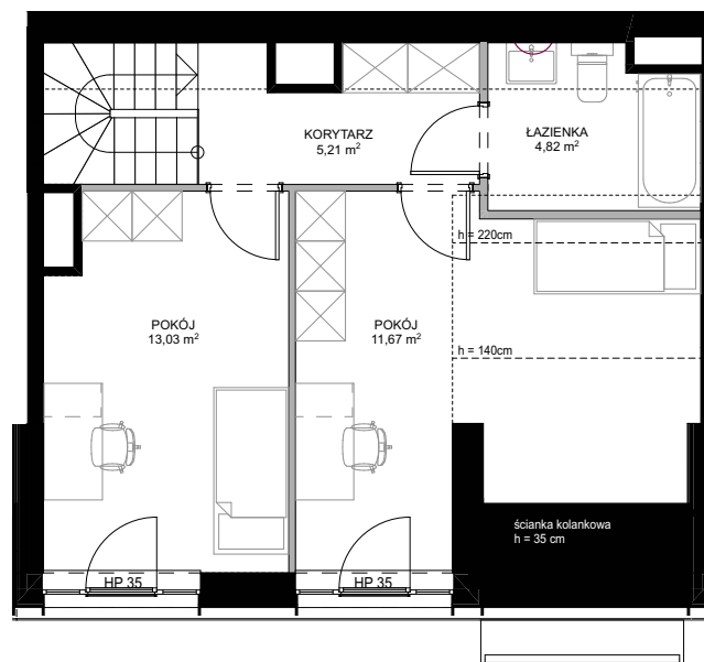
kondygnacja K4
