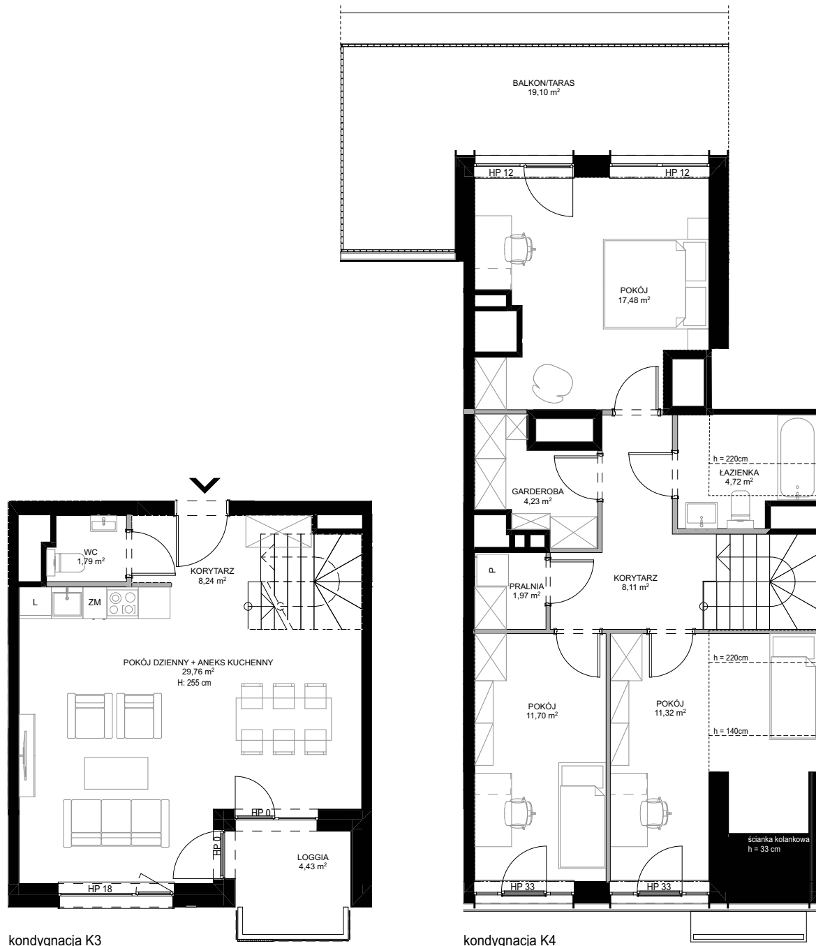
kondygnacja K3
